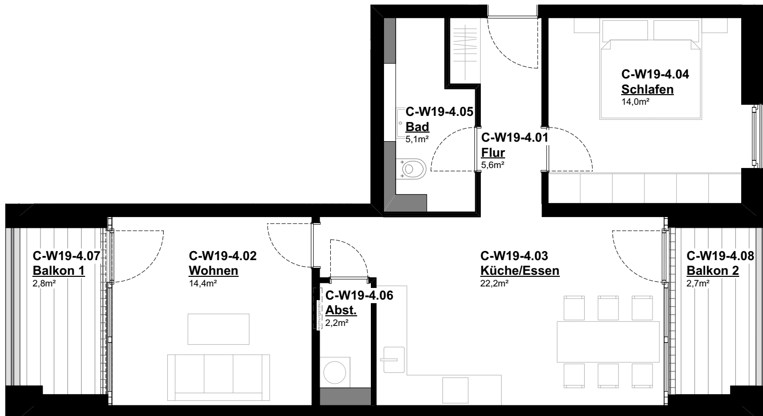
Wohnung 19 2 Zimmer 69,1 m²
